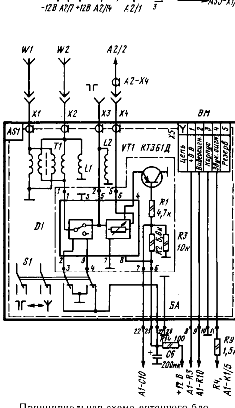
Принципиальная схема антенного блока БА телевизора «Электроника Ц-430»
