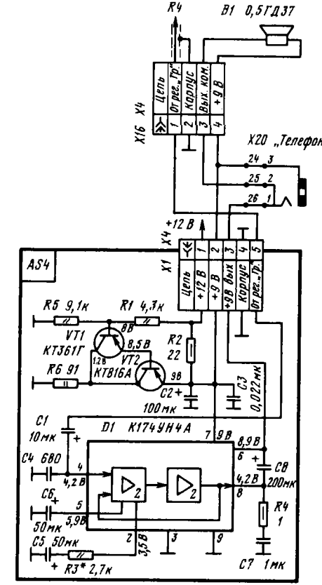
схема блока УЗ3
