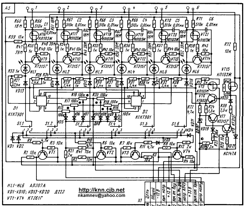
схема сенсорного устройства УС-1 телевизора «Электроника Ц-430»
