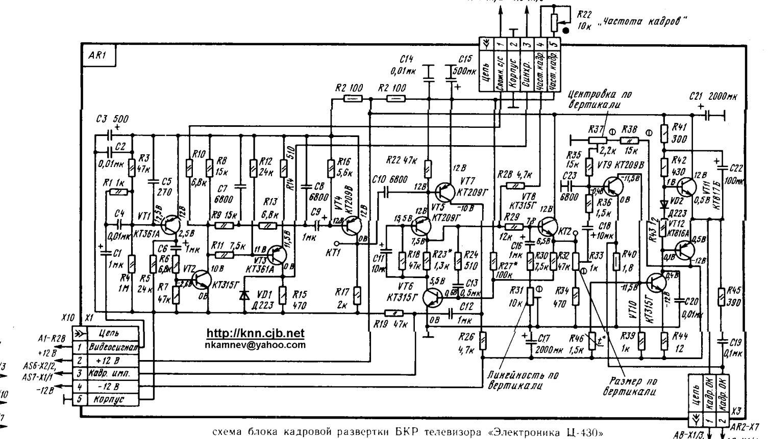
схема блока кадровой развертки БКР телевизора «Электроника Ц-430»
