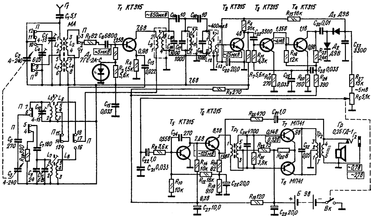
Принципиальная электрическая схема радиоприемника «Селга-402» (переключатель диапазонов в положении СВ).
