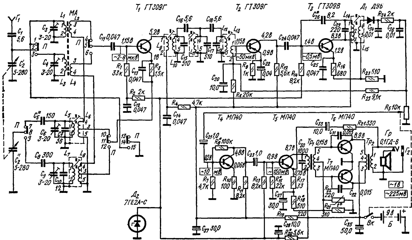
радиоприемник «Кварц-401» (переключатель диапазонов в положении ДВ).
