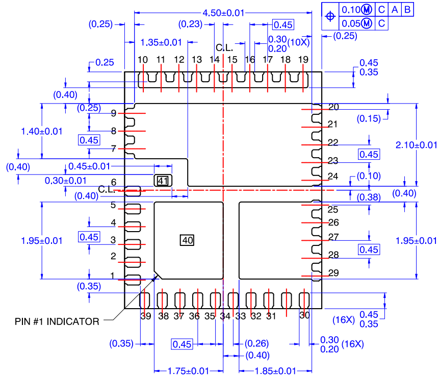
BOTTOM VIEW SCALE: 2:1
