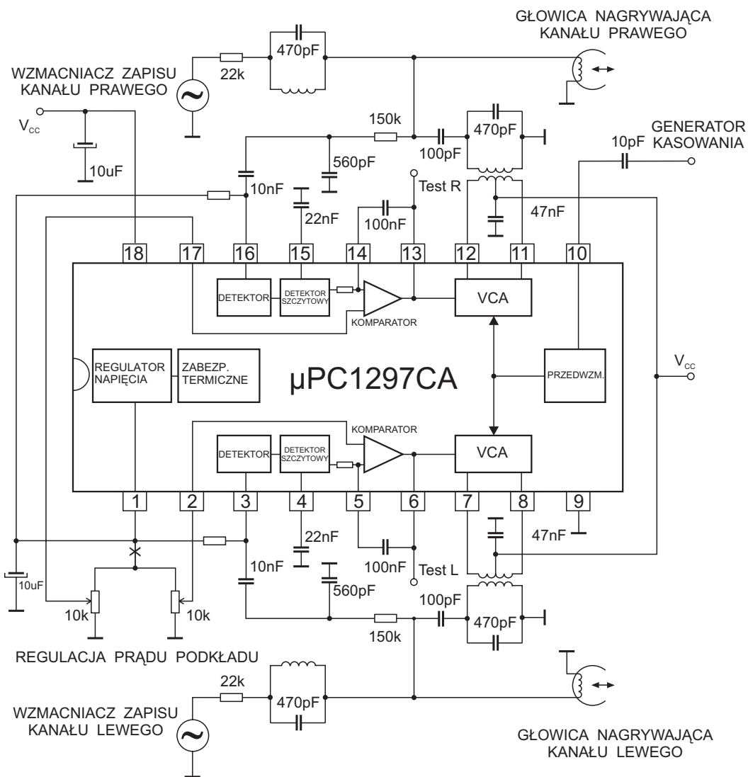
Rys.7. Schemat aplikacyjny układu scalonego \mu\text{PC1297CA} .
