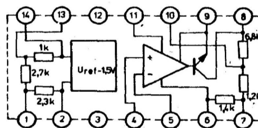
Schemat wewnętrzny
