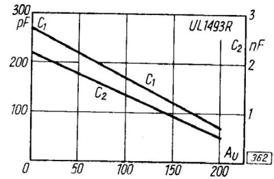
Pojemności C_1 i C_2 w funkcji wzmacnienia napięciowego
