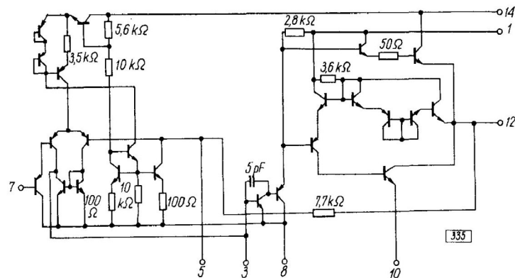
Schemat elektryczny
