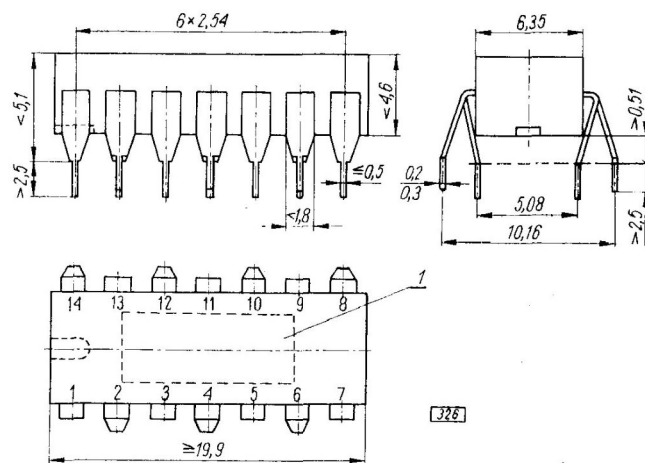
Układ scalony w obudowie typu CE75B (CB-108) 1 — płytki radiatora
