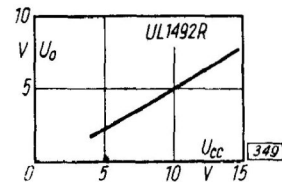
Napięcie spoczynkowe wyjściowe w funkcji napięcia zasilania
