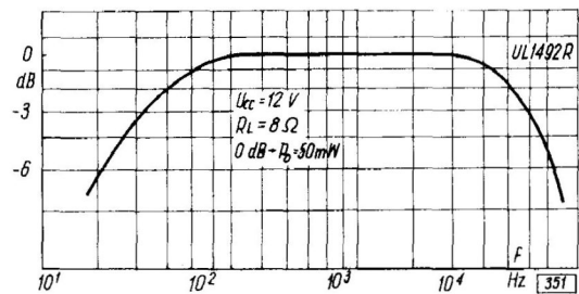
Wzmocnienie napięciowe w funkcji częstotliwości
