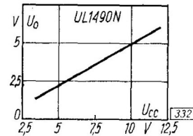
Napięcie spoczynkowe wyjściowe w funkcji napięcia zasilania
