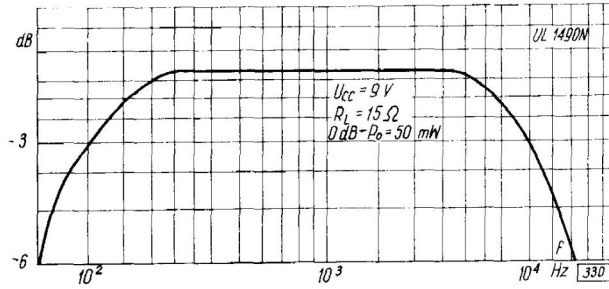
Wzmocnienie napięciowe w funkcji częstotliwości
