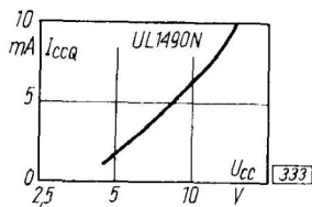
Prąd spoczynkowy zasilania w funkcji napięcia zasilania
