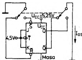
Układ pomiarowy 13. Pomiaru I_{OS}
