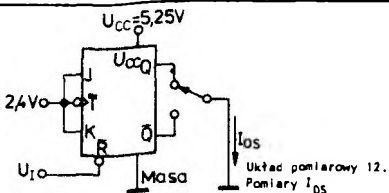
Układ pomiarowy 12. Pomiar I_{OS} Uwagi: 1. Każdy przerzutnik jest badany oddzielnie 2. W czasie pomiaru I_{OS} z wyjścia \bar{Q} wejście \bar{R} dotknąć do masy. 3. W czasie pomiaru I_{OS} z wyjścia Q przyłożyć do wejścia \bar{R} napięcie U_1 = 2,4\text{ V} wyjście \bar{Q} dotknąć chwilowo do masy.
