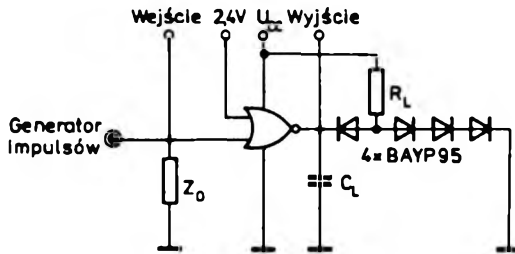
Układ pomiarowy N. Pomiar parametrów dynamicznych
