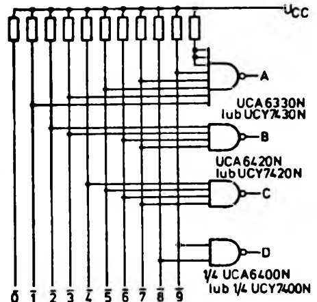
Rys. 2.19. Schemat ideowy koderu kodu dziesiętnego (1 z 10) na kod BCD 8421.
