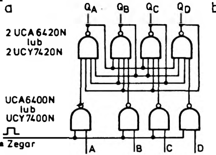
Rys. 2.18. Synchroniczny przerzutnik czterowejściowy a — schemat logiczny, b — tabela stanów
