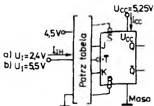
Układ pomiarowy 11. Pomiar I_{IH} , I_{OC}
