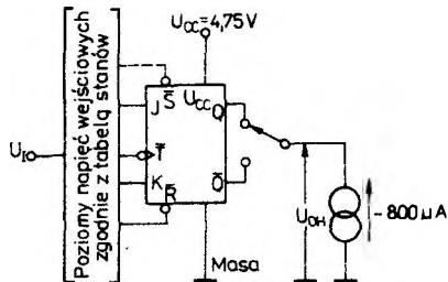
Każdy przerzutnik jest badany oddzielnie. Układ pomiarowy 9. Pomiar U_{0H}
