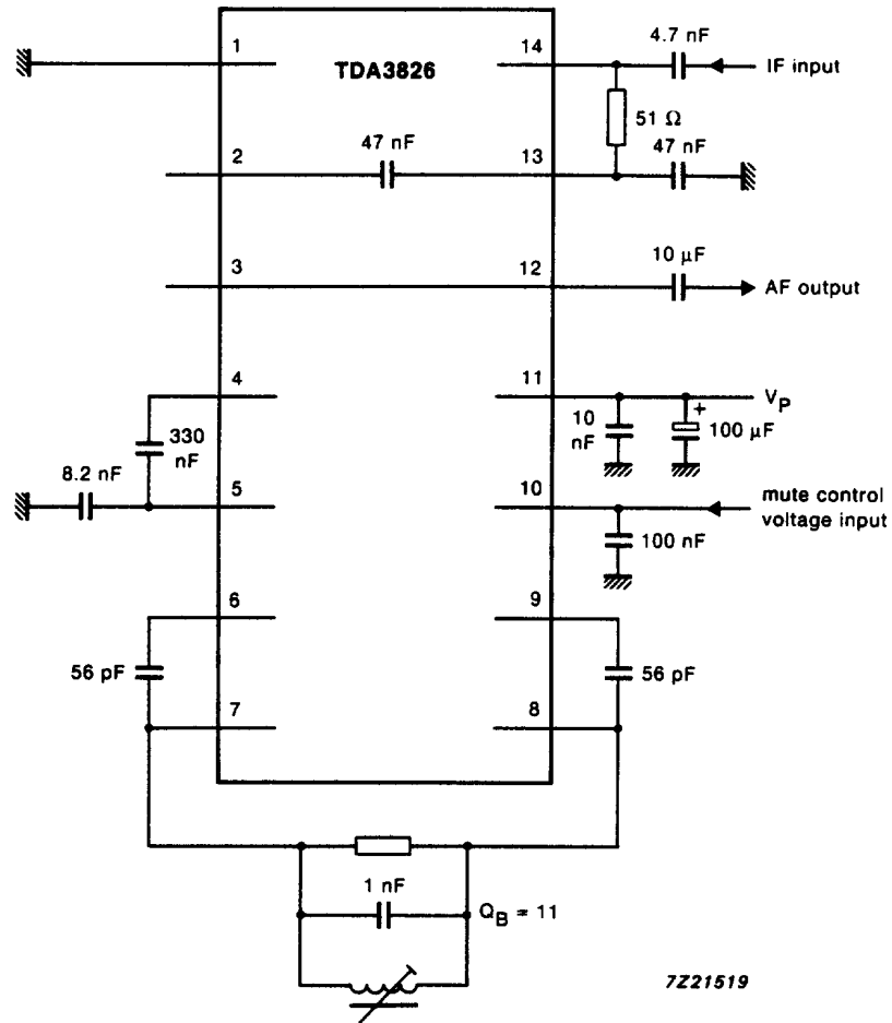
Fig.2 Test circuit.
