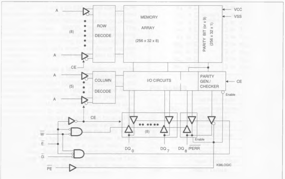
BLOCK DIAGRAM N° 2
