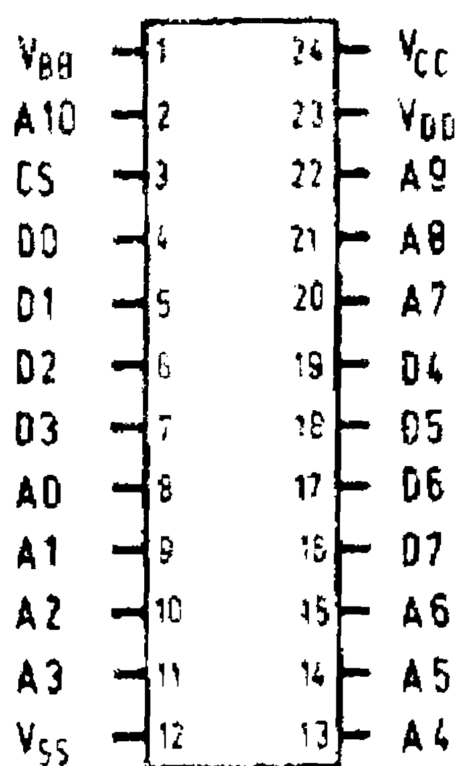
MCM 6590, 6591 (2 KByte)
