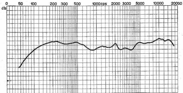
Charakterystyka skuteczności mikrofonu MDO-VIII
